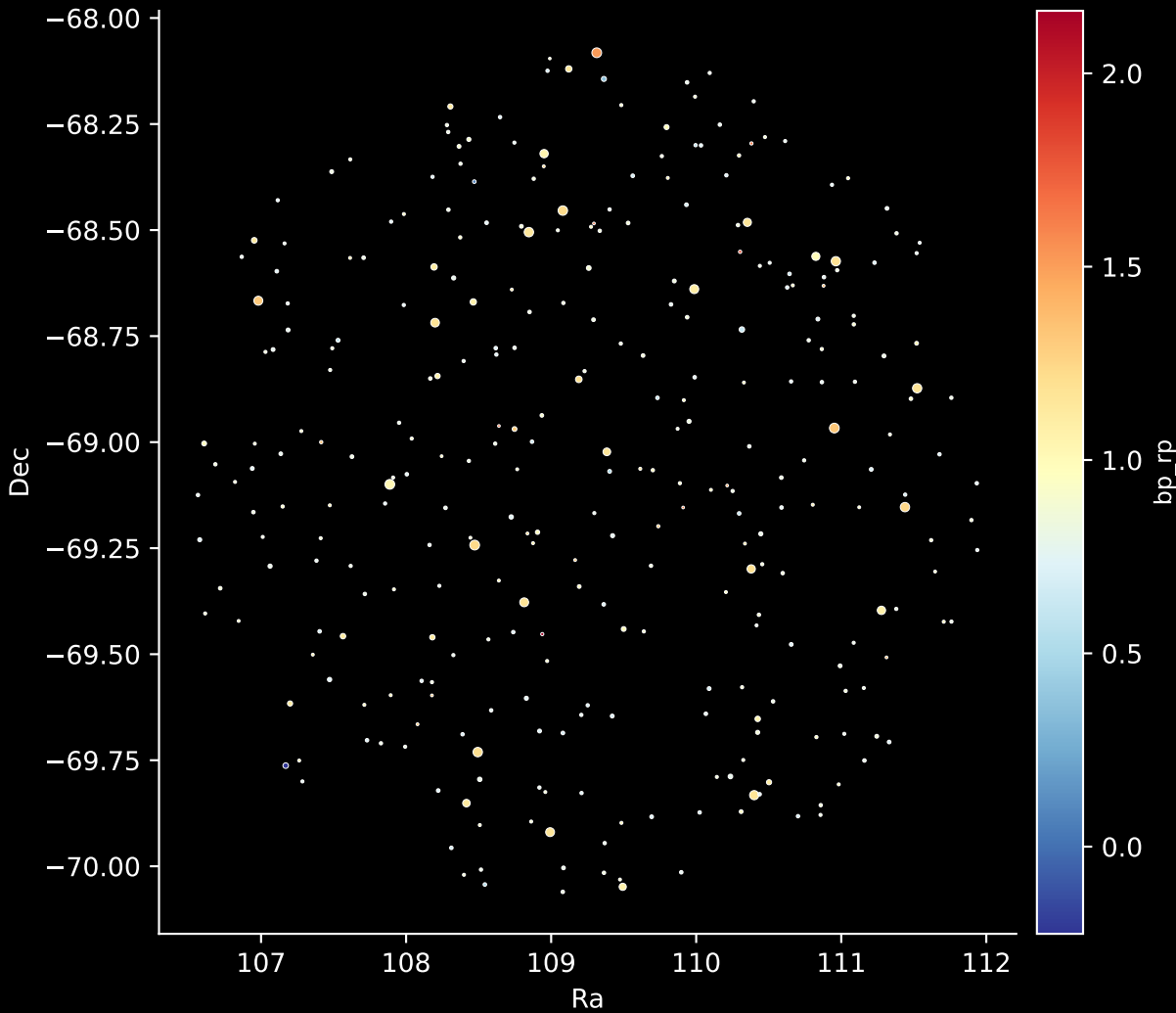
GALAH DR4 Field: [7047] Stars: 311
