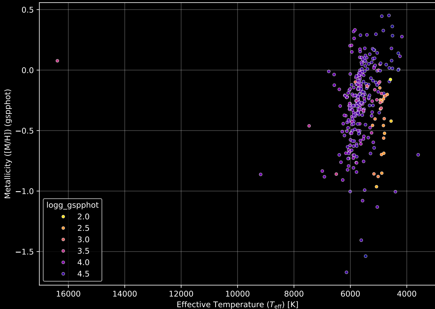
GALAH DR4 Field: [7047] Stellar Population Parameters (n= 311)
